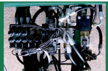
Auf Wunsch: Elektro-hydr. Steuerblock im Rebenladewagen integriert
